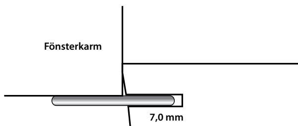
Montage med plastclips
