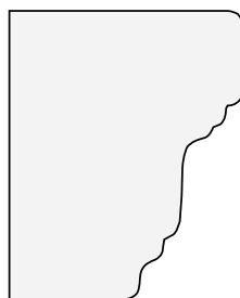
Fönsterbänklister Profilnummer 20 45 x 57
