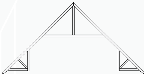
Svensk takstol
