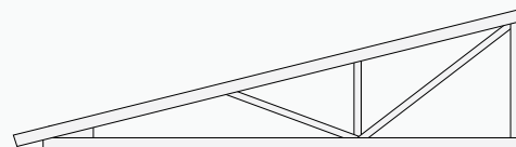
Pulpettakstol
